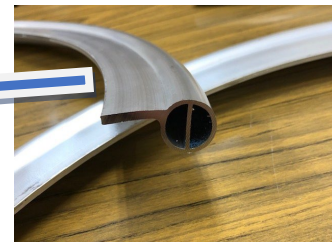
開発したハンドリムの断面
