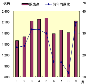
半導体販売高
